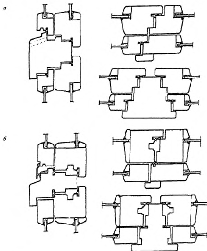
a – вариант конструкции с распашным открыванием створок, с двумя контурами прокладок в наружной и внутренней створках; b – вариант конструкции с поворотно-откидным открыванием створок, с двумя контурами прокладок во внутренней створке и коробке, с алюминиевым дождезащитным профилем
