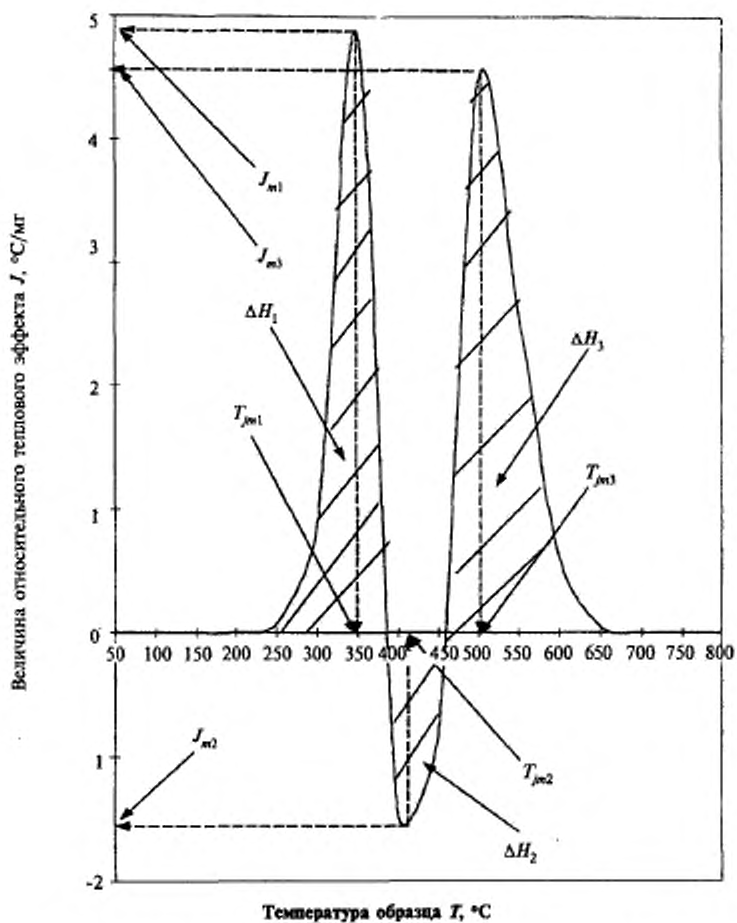
Рисунок А.3 — Пример определения значений относительного теплового эффекта по ДТА-зависимости
