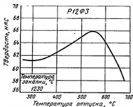
Черт. 8
