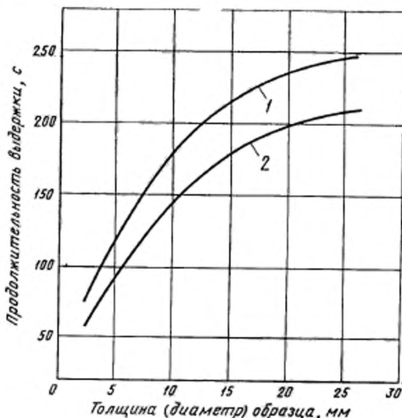
Черт. 1
