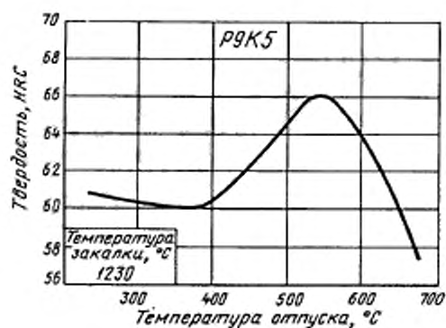
Черт. 10
