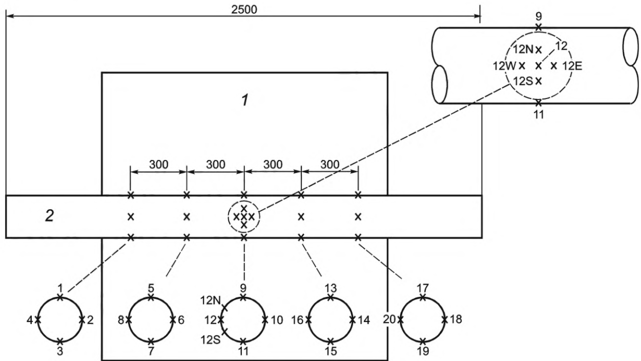
1 — климатическая камера; 2 — держатель образца
