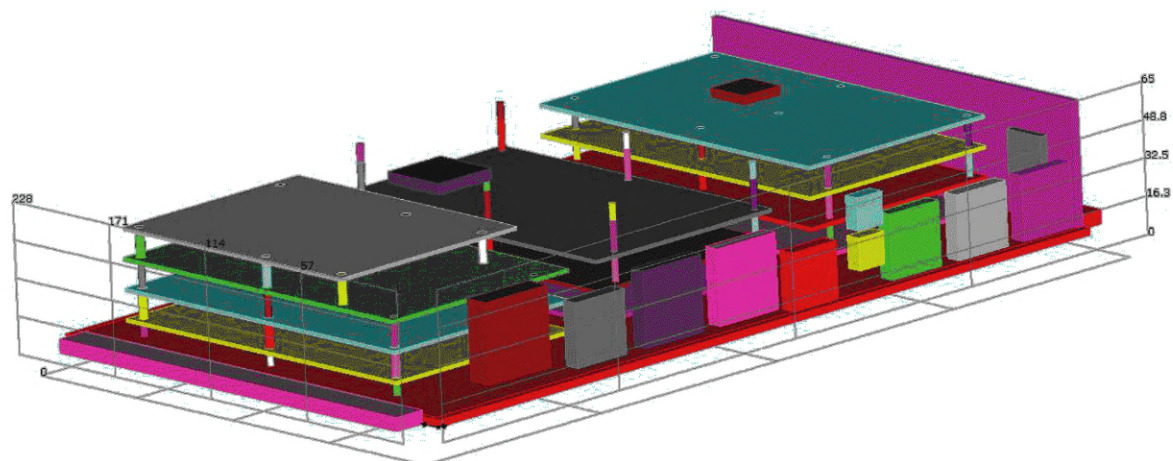
Рисунок А.1 — Конструкция блока ЭА, импортированная из CAD-системы в подсистему АСОНИКА-М-3D
