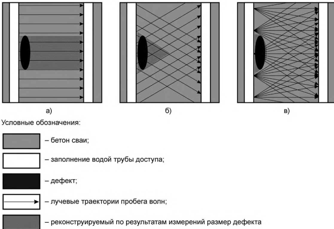
Рисунок 7.1 — Условная схема локализации дефекта при использовании: стандартной методики измерений (а); дополнительных измерений по методике косых прозвучиваний (б); измерений по томографической методике (в)
