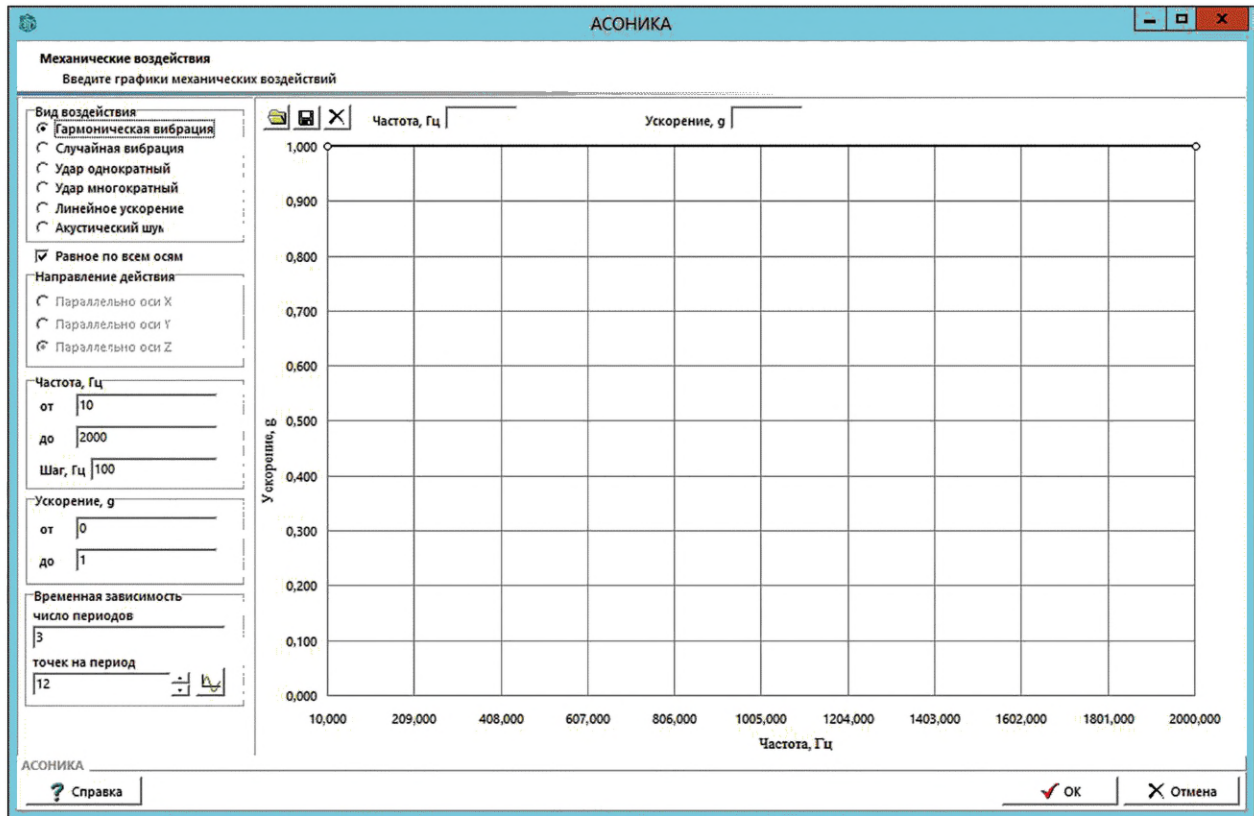
Рисунок А.5 — График зависимости амплитуды входного ускорения синусоидальной вибрации от частоты
