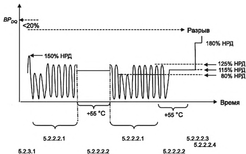
Рисунок 4 — Проверка ожидаемых эксплуатационных характеристик хранилища сжатого водорода
