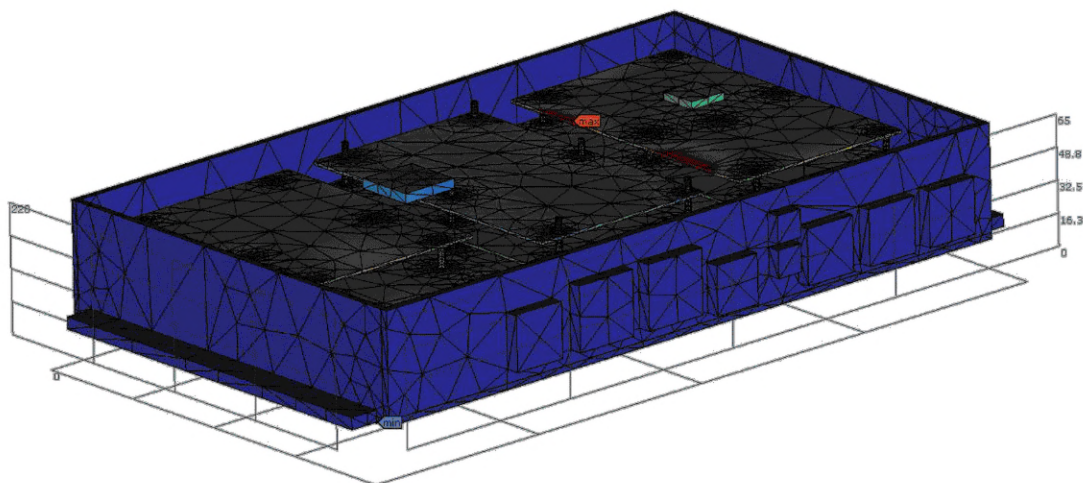
Рисунок А.7 — Среднеквадратические суммарные ускорения во всех точках конструкции блока ЭА
