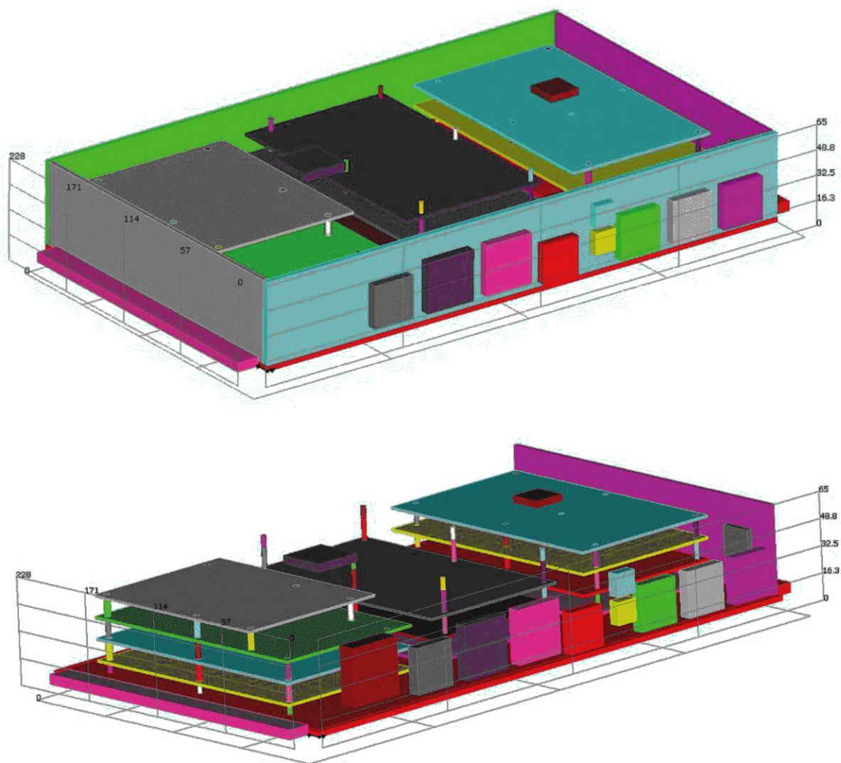
Рисунок А.4 — Конструкция блока ЭА, импортированная из САD-системы в подсистему АСОНИКА-М-3D
