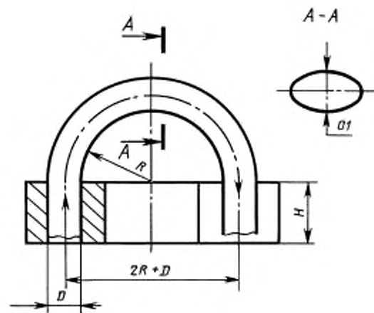
R — минимально допустимый радиус изгиба рукава; D — диаметр рукава; H — высота приспособления, не менее наружного диаметра рукава
