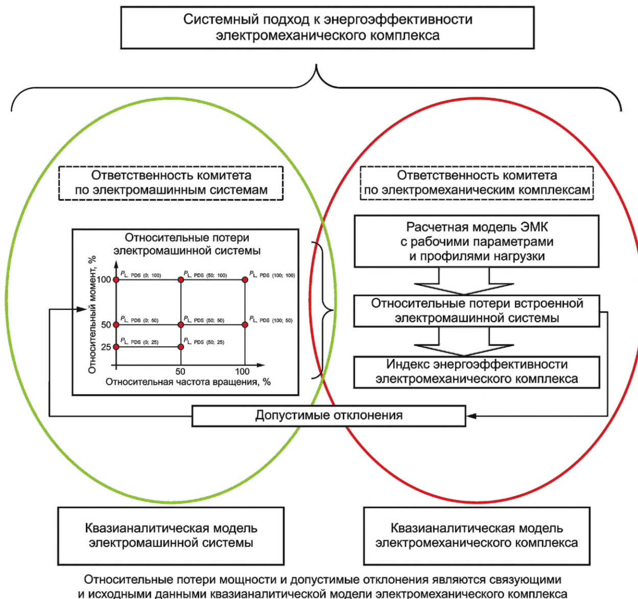
Рисунок 6 — Ответственность и процедуры при определении индекса энергоэффективности электроμηχανического комплекса
