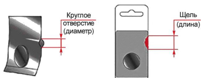
Рисунок Е.5 — Допускаемые отверстия в упаковке
