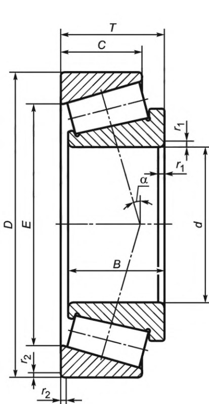
Рисунок 1 — Конструктивные исполнения 00, 02
