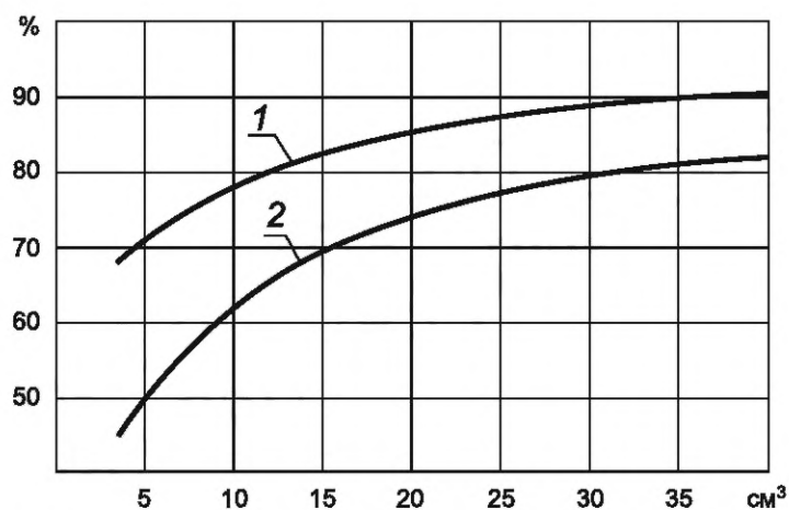
Рисунок 1 — Зависимость минимально допустимого значения коэффициента подачи и общего КПД пластинчатых насосов от рабочего объема в диапазоне от 3,2 до 40,0 см 3
