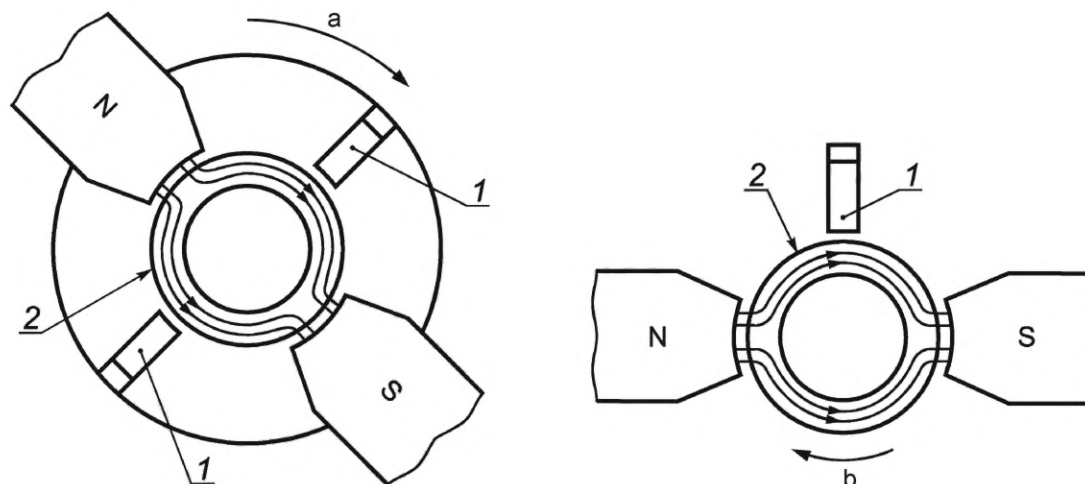
а) Способ вращающегося магнитного преобразователя — продольное перемещение трубы б) Способ неподвижного магнитного преобразователя — вращательно-поступательное движение трубы
