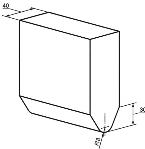
Рисунок 2 — Размеры ударника
