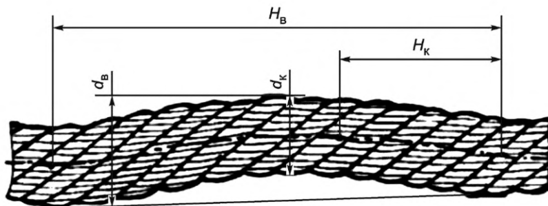
Рисунок А.5 — Волнистость несущего каната
