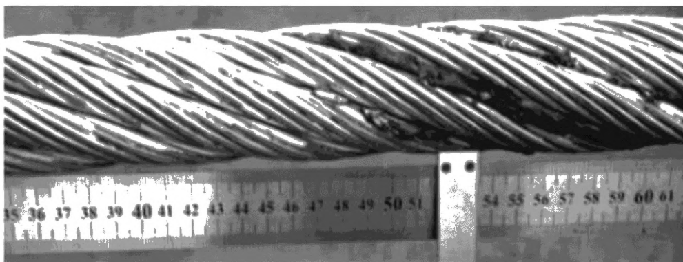
Рисунок А.5 — Волнистость несущего каната
