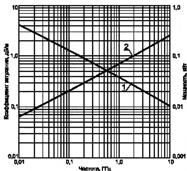
Частотные зависимости
