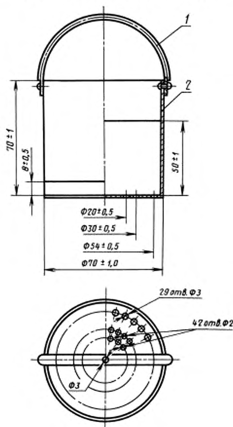
1 — ручка; 2 — корпус
