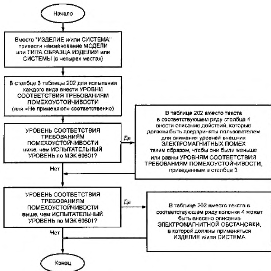
Рисунок 203 — Порядок заполнения таблицы 202 [см. 6.8.3.201, перечисление а) 6)]
