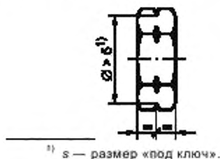
Рисунок 6 — Альтернативная маркировка левой резьбы
