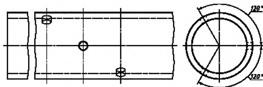
Рисунок В.1 — Эталонный образец с тремя отверстиями
