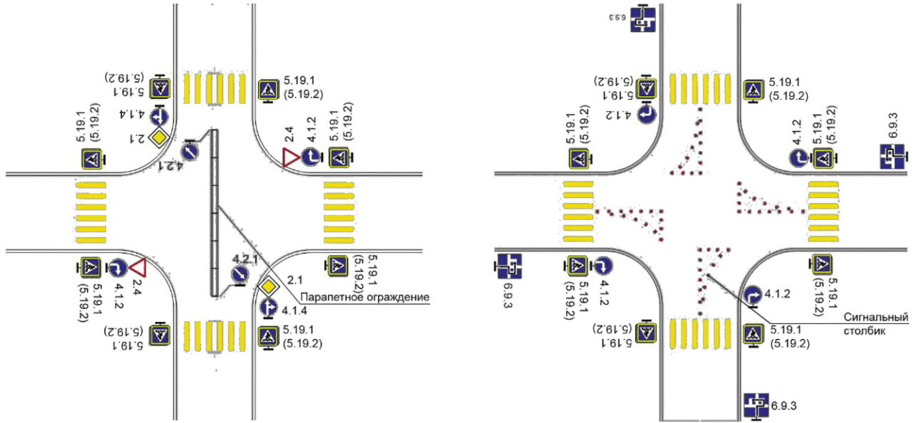
г) Перекрытие сквозного движения при помощи параллельного ограждения
