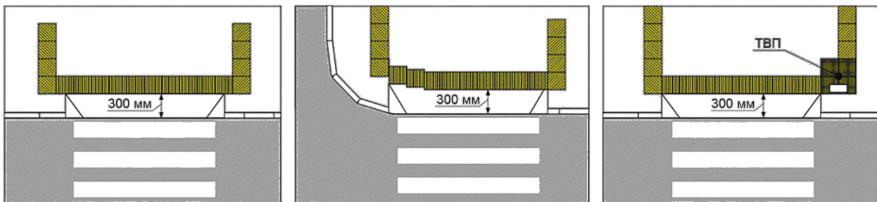
а), б) На нерегулируемых пешеходных переходах
