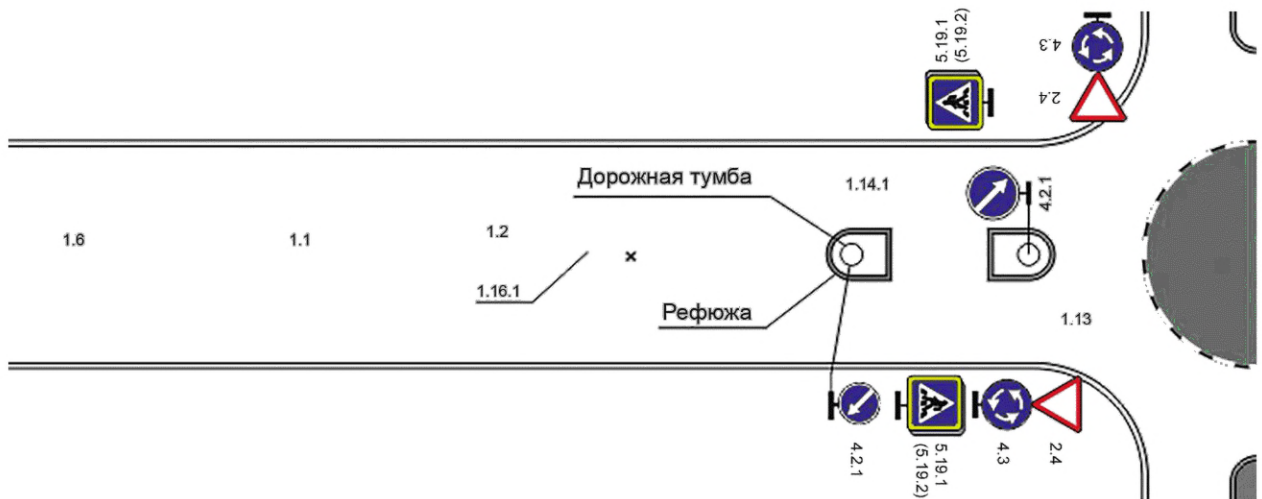
Рисунок Б.16 — Пример обустройства кольцевого пересечения пешеходными переходами и техническими средствами организации дорожного движения
