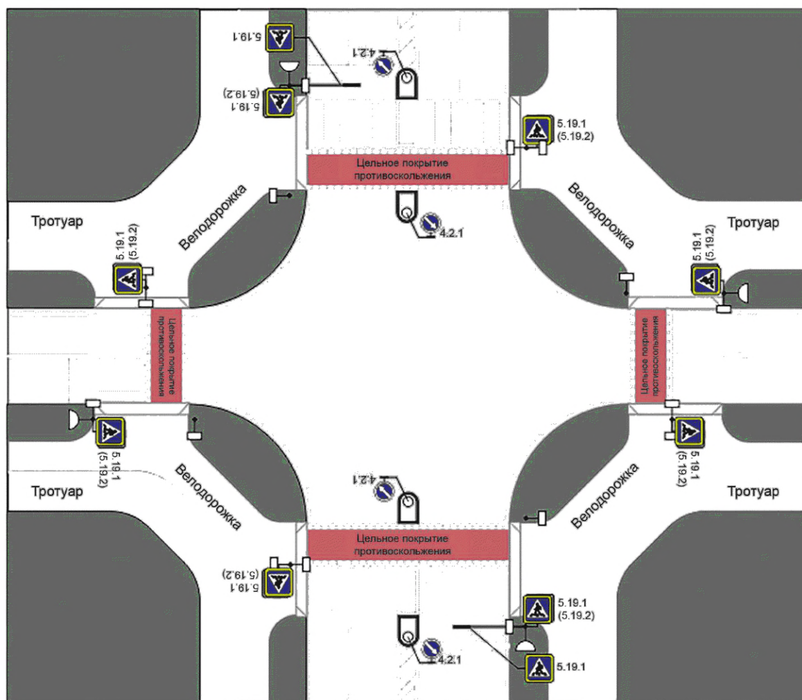
Рисунок Б.28 — Организация пересечения велосипедной дорожки с проезжей частью, смежной с пешеходным переходом
