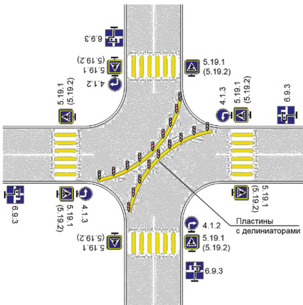
б) Установка delineаторов и дорожных пластин
