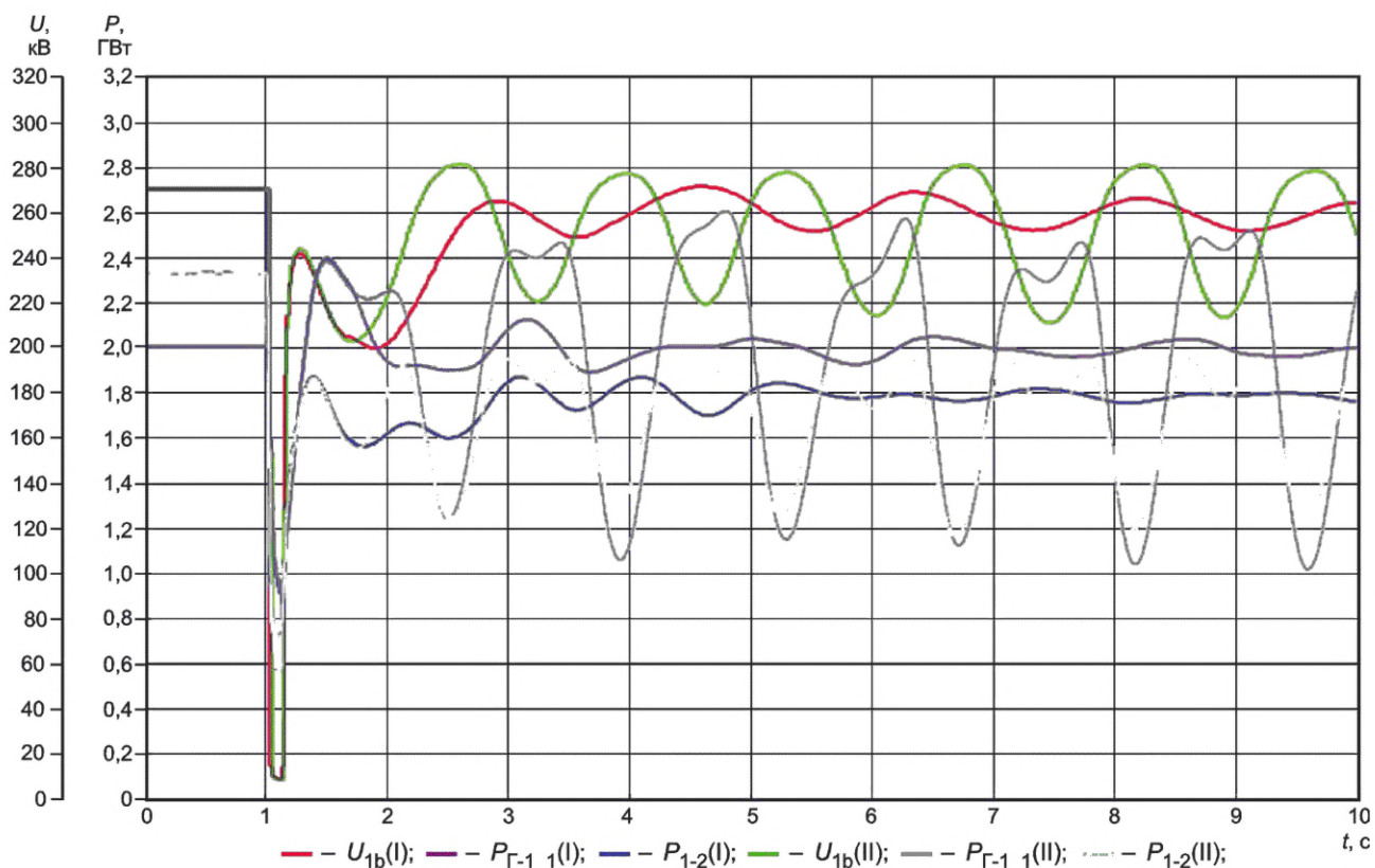
Рисунок Д.29 — Корректная работа функции блокировки каналов стабилизации (системного стабилизатора) при аварийном отключении генератора на электрической станции № 2
