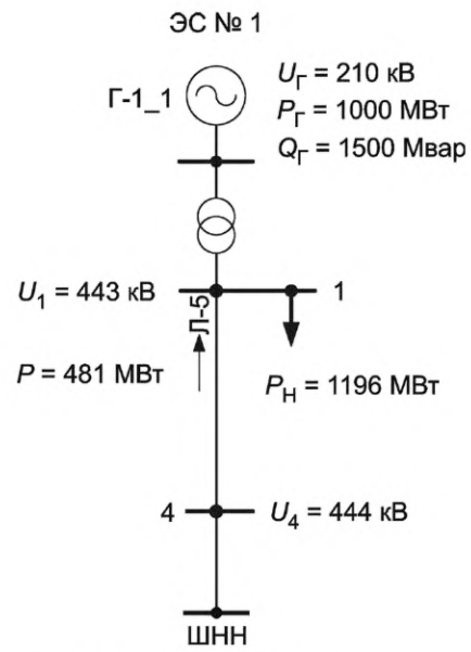
Рисунок Д.2 — Схема 1. Режим 2
