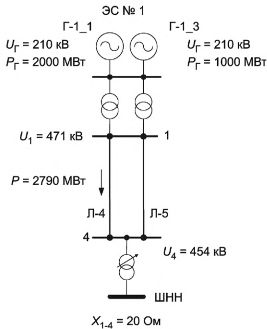
Рисунок Г.20 — Схема 7. Режим 17
