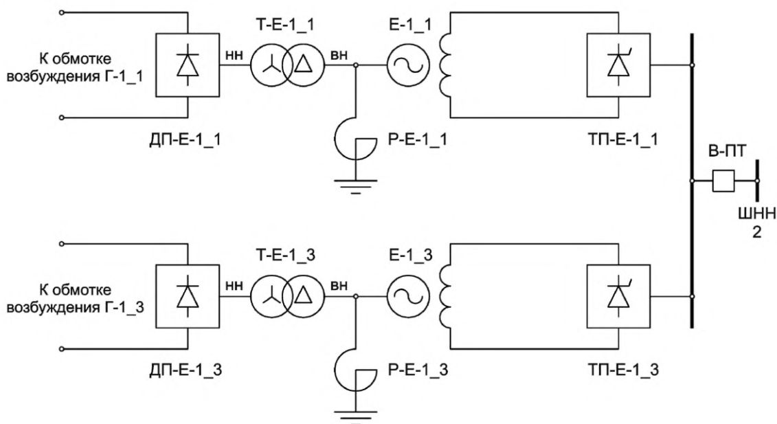
ТП-Е-1_1 и ТП-Е-1_3 — тиристорные преобразователи; ДП-Е-1_1 и ДП-Е-1_3 — диодные преобразователи; Р-Е-1_1 и Р-Е-1_3 — реакторы; Т-Е-1_1 и Т-Е-1_3 — согласующие трансформаторы
