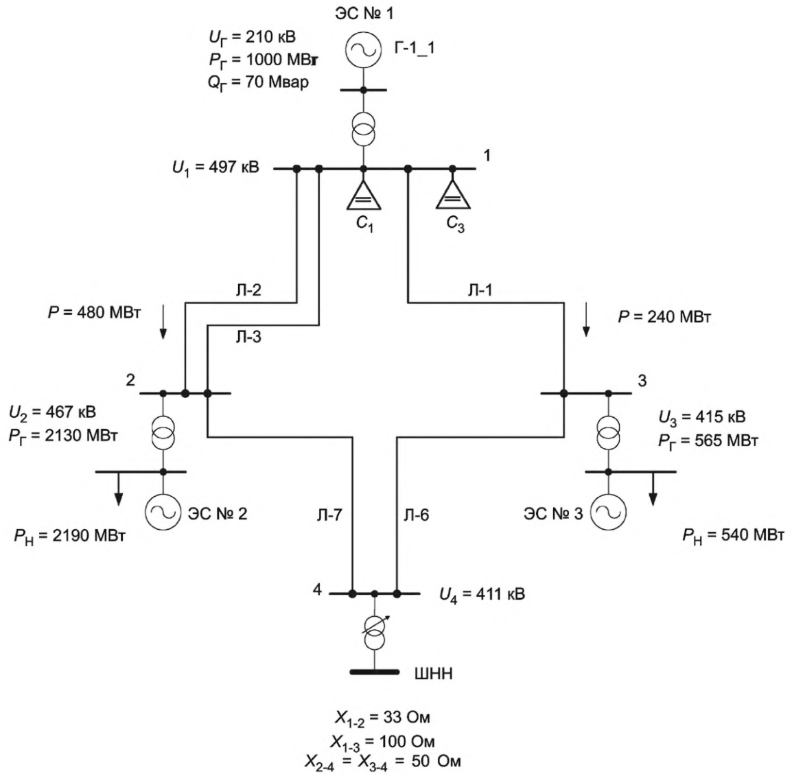
Рисунок Г.17 — Схема 3. Режим 14
