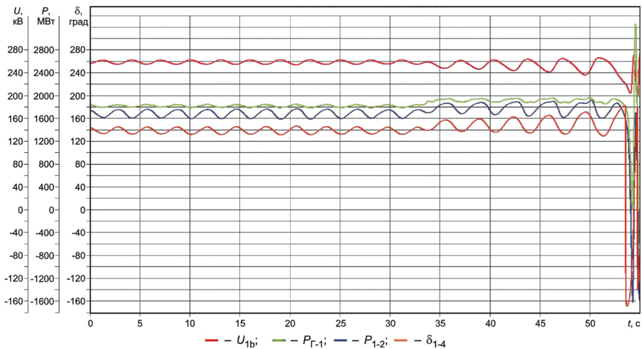
б) Неэффeктивная работа каналов стабилизации
