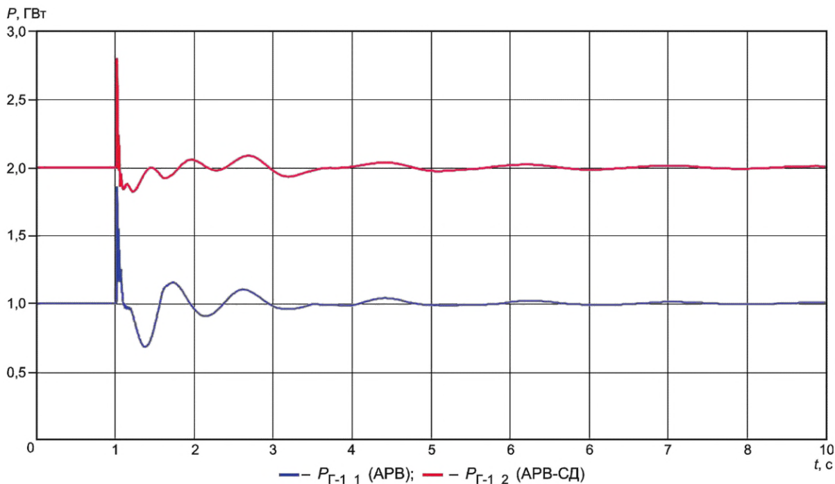
Рисунок Д.25 — Корректная работа АРВ сильного действия при совместной работе с регуляторами других типов на одной электростанции
