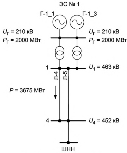
Рисунок Д.17 — Схема 7. Режим 16
