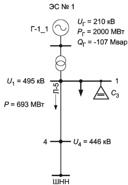
Рисунок Д.3 — Схема 1. Режим 3
