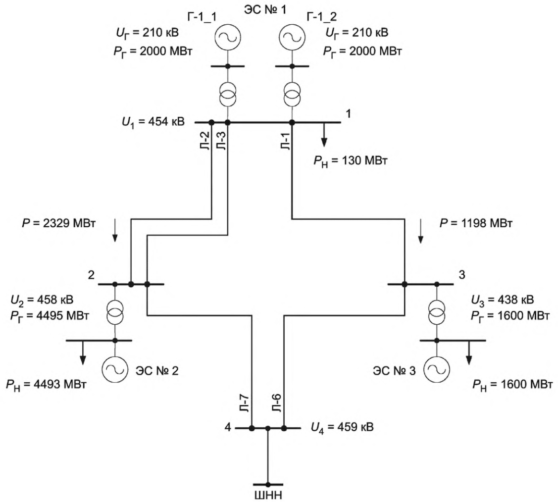
Рисунок Д.6 — Схема 3. Режим 5
