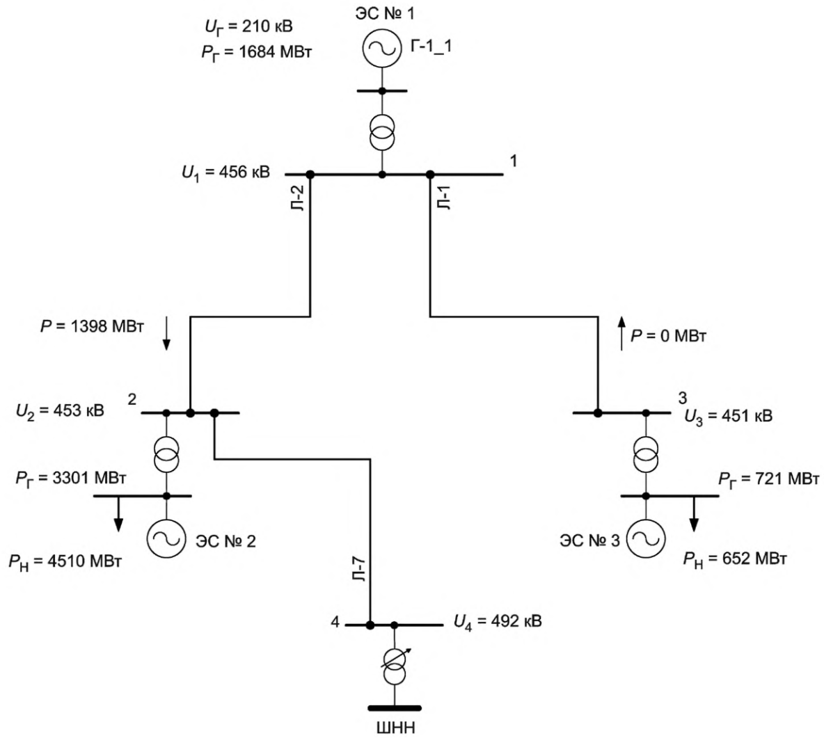
Рисунок Д.5 — Схема 2.2. Режим 4
