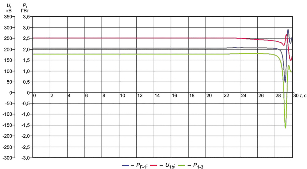
а) Эффективная работа каналов стабилизации
