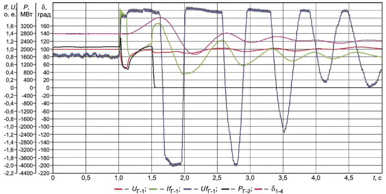
Рисунок Г.31 — Корректная работа АРВ сильного действия с учетом работы устройств ПА
