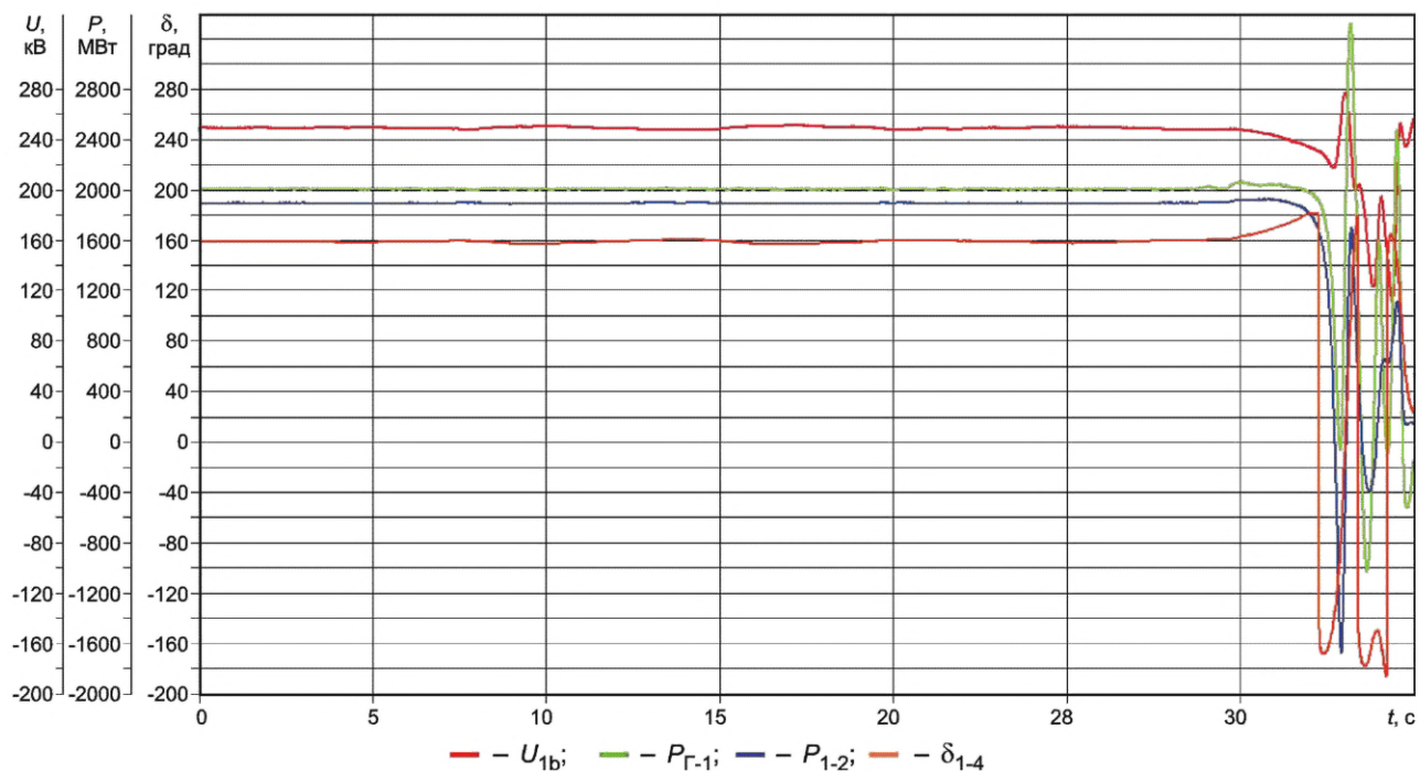
а) Эффeктивная работа каналов стабилизации
