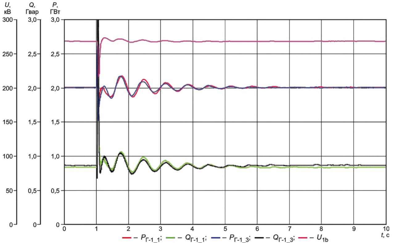
Рисунок Д.41 — Корректная работа АРВ сильного действия при однофазном КЗ на шинах электрической станции № 1 при совместной работе двух регуляторов в составе укрупненного блока синхронных генераторов
