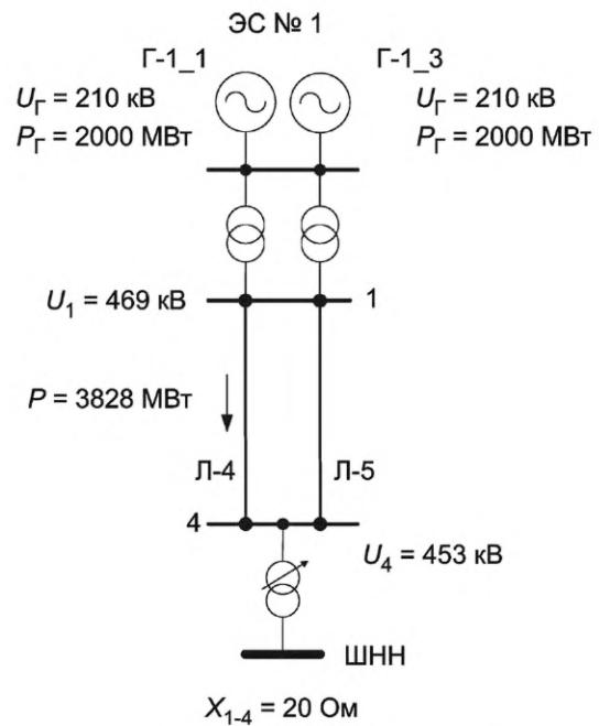
Рисунок Г.19 — Схема 7. Режим 16
