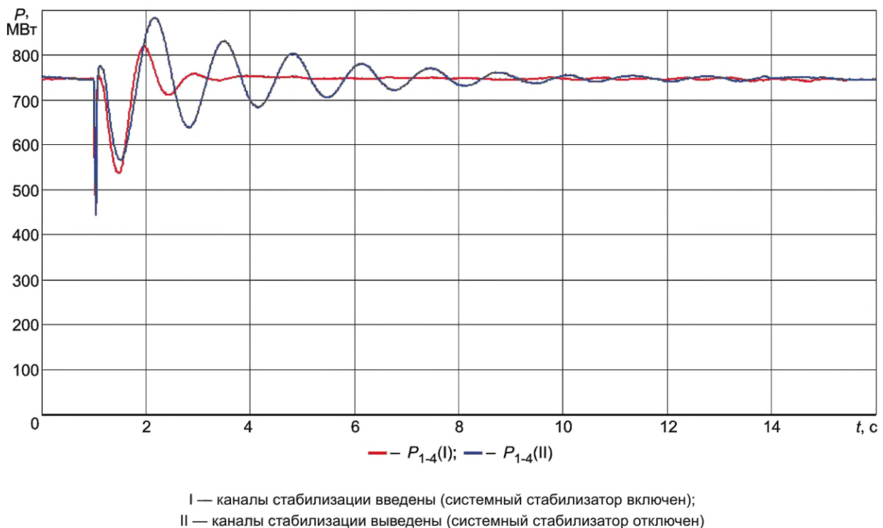
Рисунок Г.21 — Эффективная работа каналов стабилизации (системного стабилизатора)
