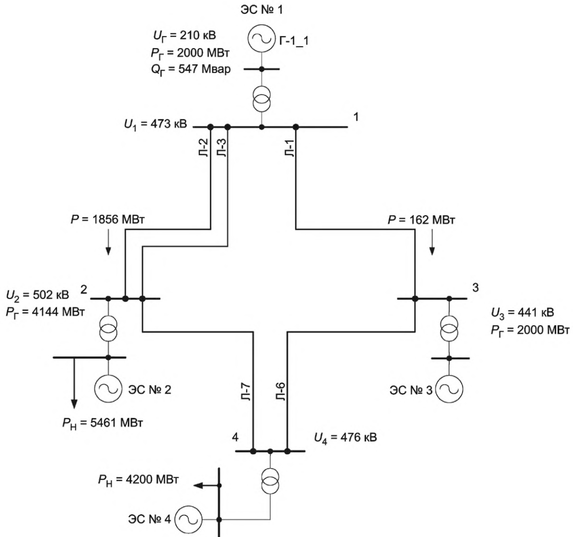
Рисунок Д.11 — Схема 4. Режим 10
