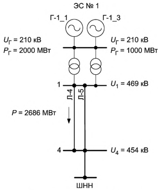
Рисунок Д.18 — Схема 7. Режим 17
