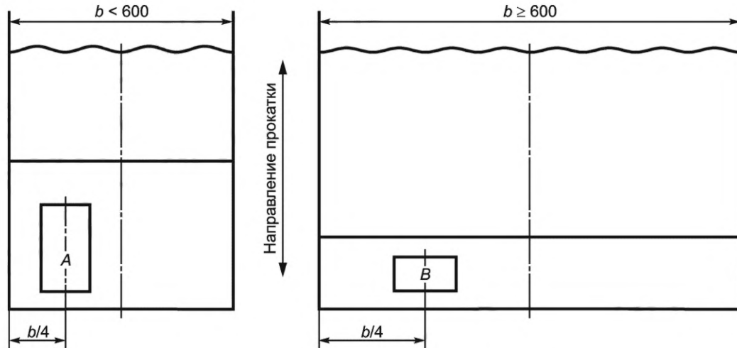
Рисунок Б.1 — Схемы отбора проб
