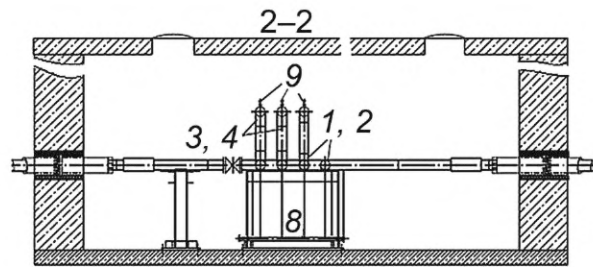
в) Вид 2-2
