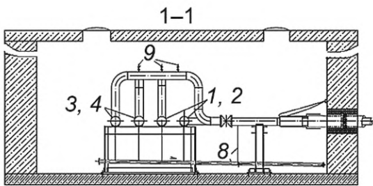
б) Вид 1-1
