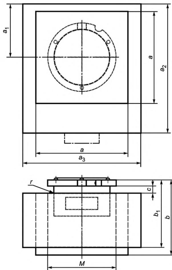
Рисунок 6 — Положение центра тяжести ламп с цоколем PK32d (заштрихованные области)
