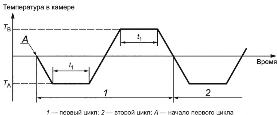
Рисунок 7 — Схема температурного цикла испытаний, приведенная в МЭК 60068-2-14, испытание Nb
