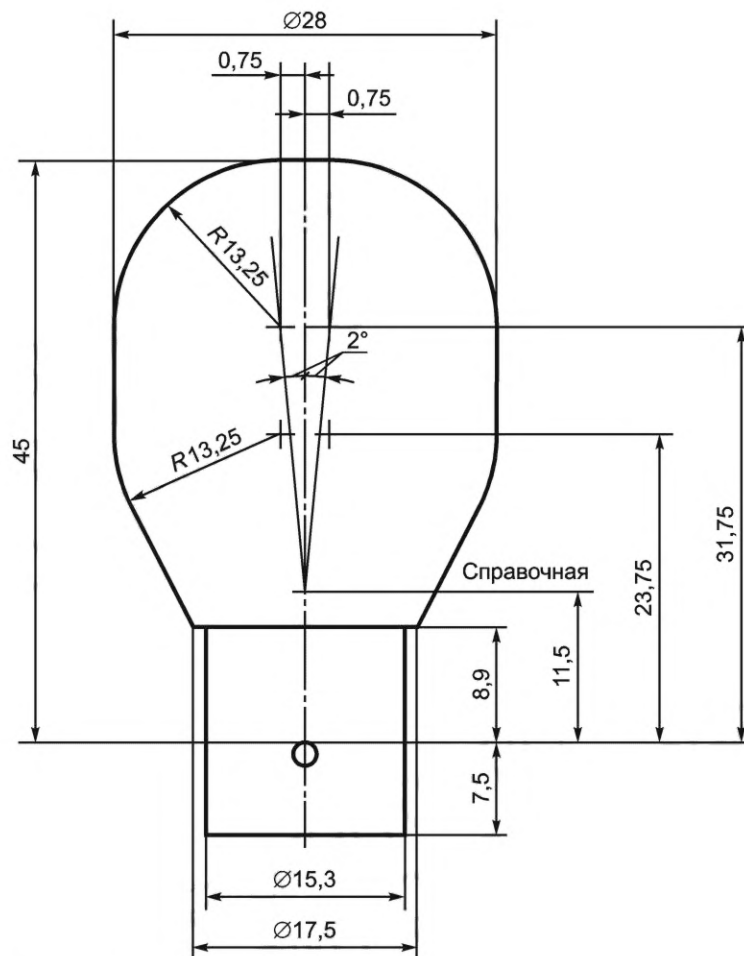
Рисунок F.5 — Максимальные контуры ламп накаливания категорий P21W, PY21W, P21/4W и P21/5W
