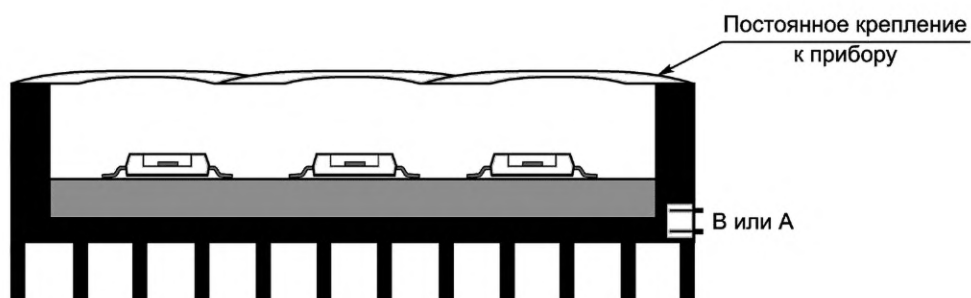
Рисунок 5 — Пример незаменяемого СД источника света
