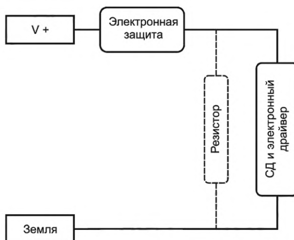
Рисунок 8 — Типичная электрическая схема СД источников света категорий LR3, LR5, LY3, LY5, LW3, LW5 и L1/6
