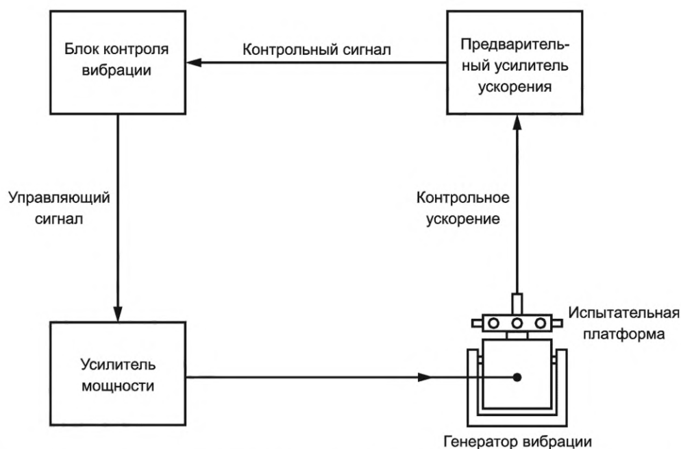
Рисунок В.1 — Рекомендуемая схема расположения оборудования для испытаний ламп на ШСВ или УСВ
