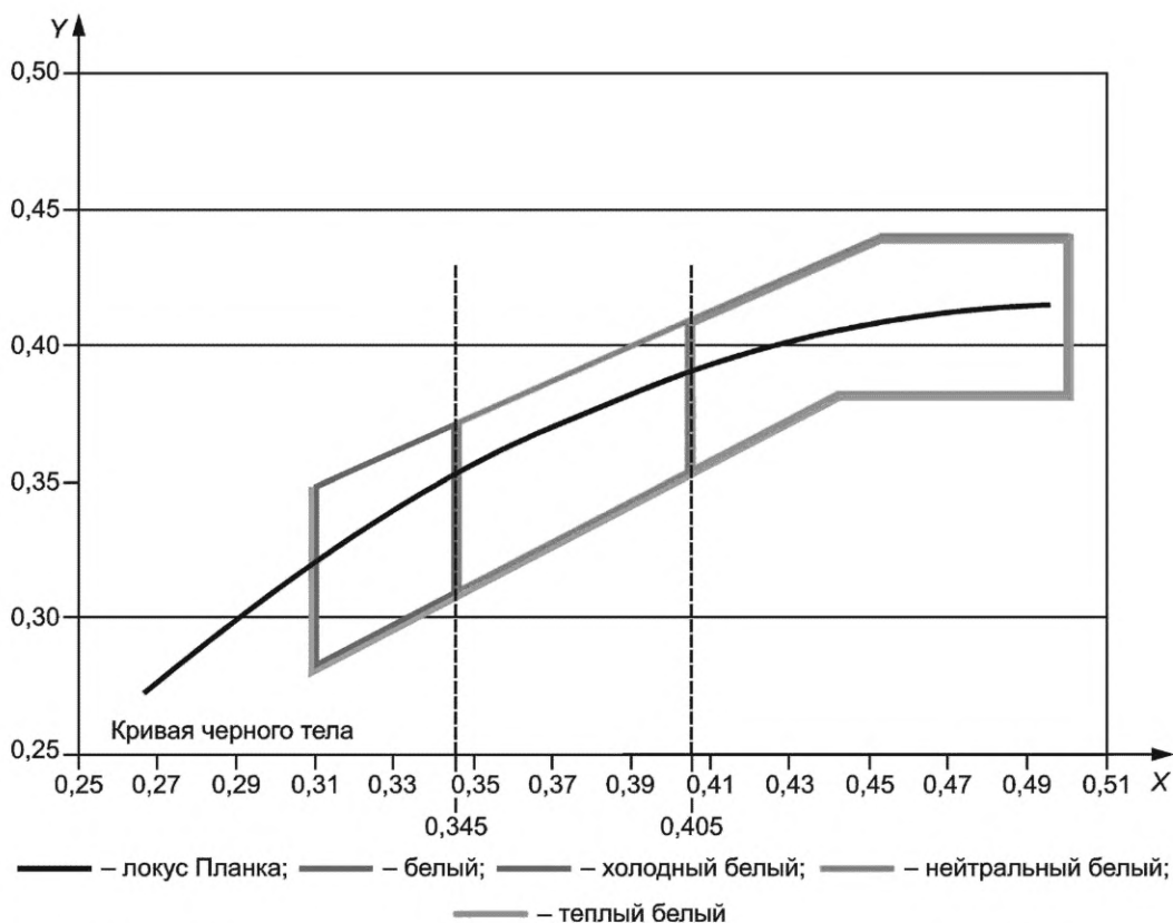
Рисунок 13* — График пространства белого цвета с тремя группами белого цвета для СД источников света
