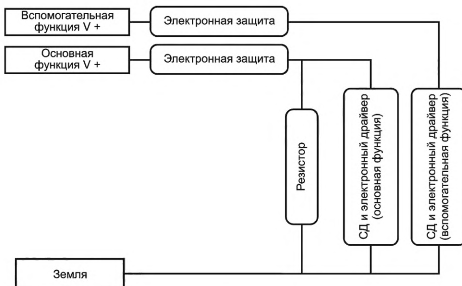
Рисунок 9 — Типичная электрическая схема СД источника света категории LR4
