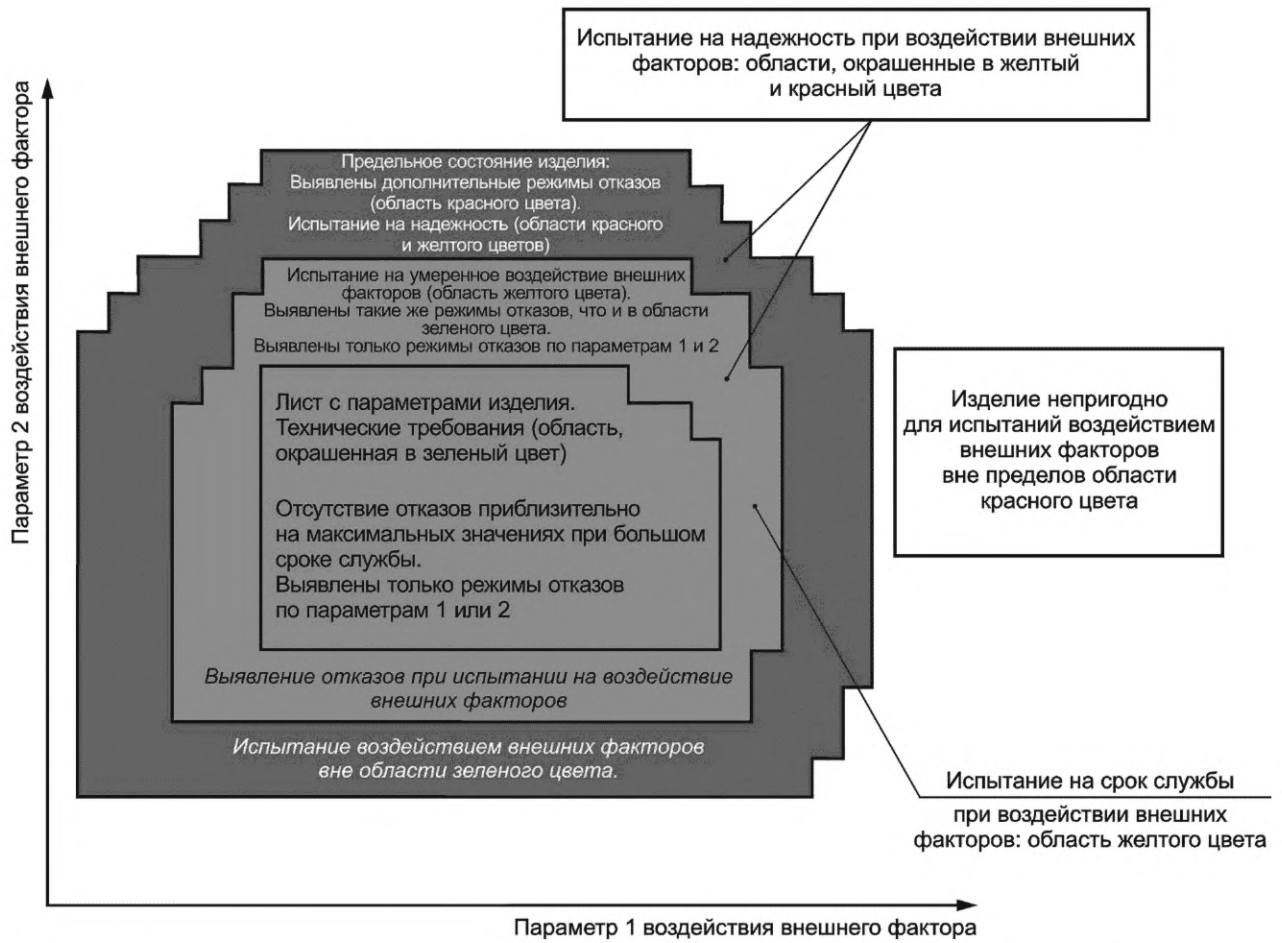
Рисунок М.1 — Схема концепции испытаний на воздействие внешних факторов по двум моделям параметров
