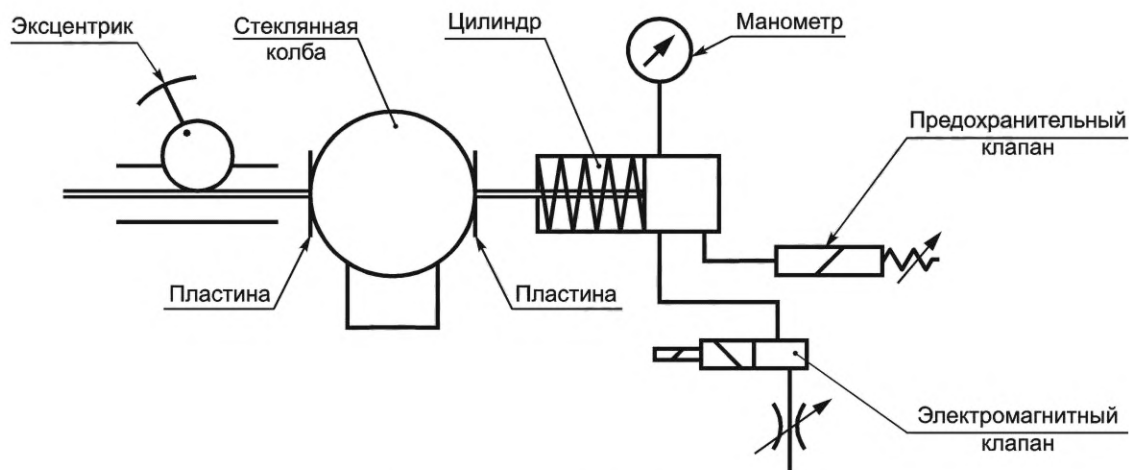
Рисунок С.1 — Схема испытательной установки
