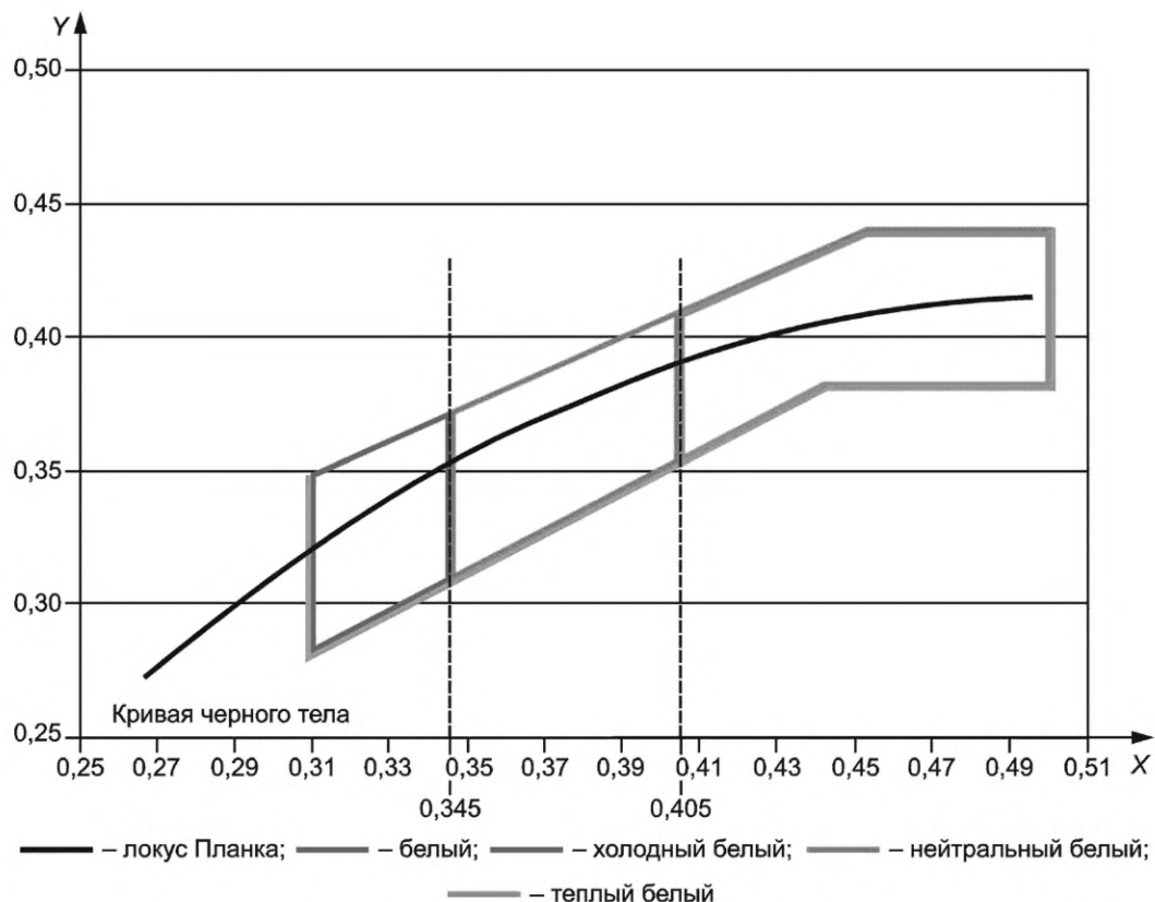
Рисунок 14* — График пространства белого цвета с тремя группами белого цвета для разрядных ламп
