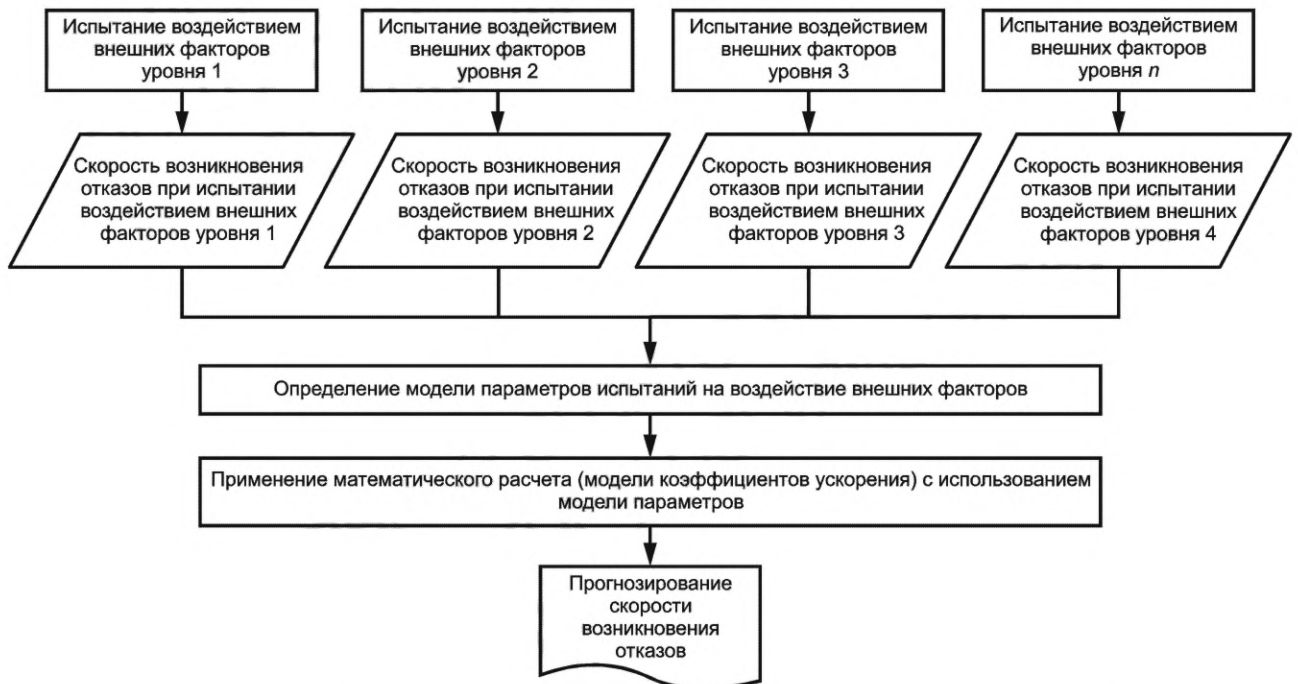
Рисунок М.2 — Блок-схема процесса подтверждения надежности корпусированных СД
