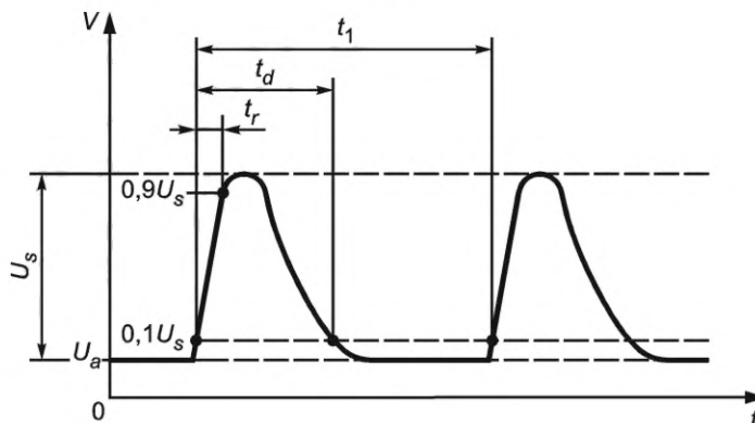
Рисунок 11 — Испытательный импульс 2а (см. ИСО 7637-2)
