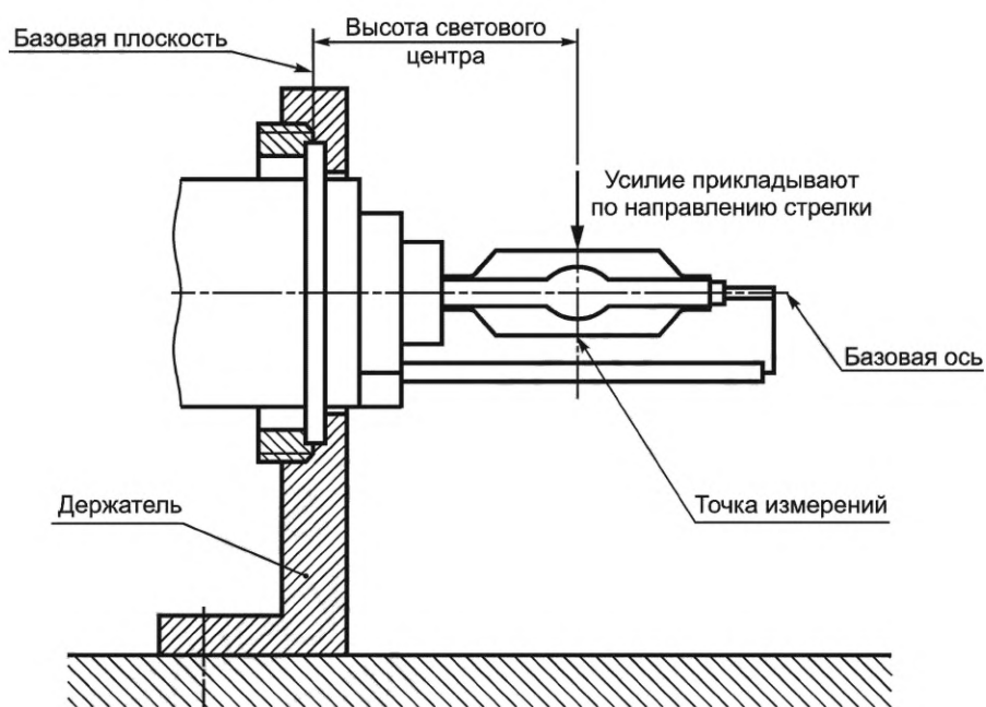
Рисунок Е.1 — Схема испытательной установки
