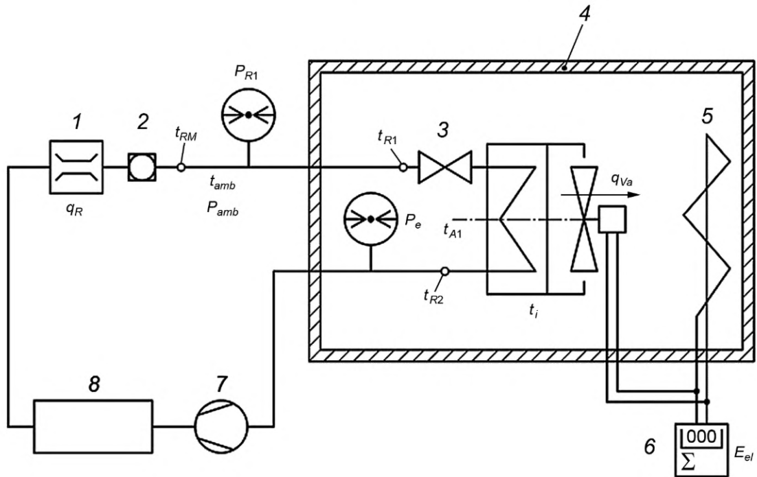
1 — расходомер хладагента; 2 — смотровое стекло; 3 — расширительное устройство; 4 — calorиметрическая комната; 5 — электронагреватель; 6 — счетчик потребления электроэнергии; 7 — компрессор; 8 — конденсатор
