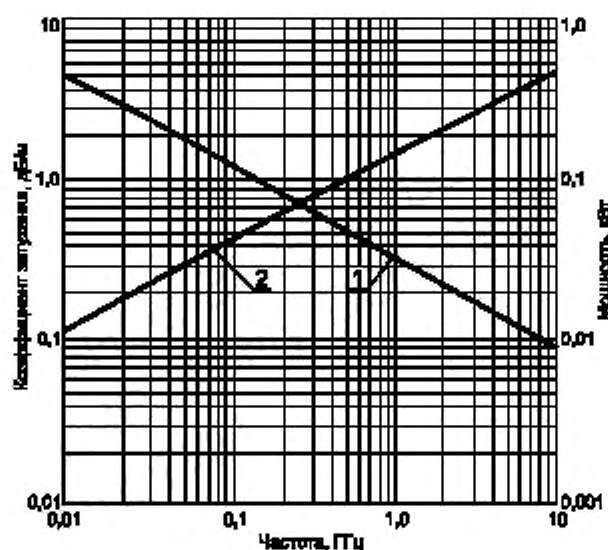
Частотные зависимости
