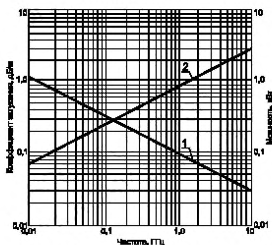
Частотные зависимости
