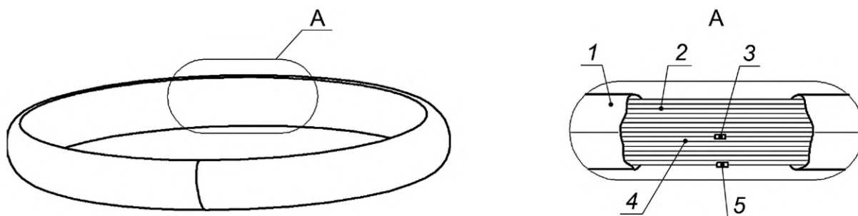
а – круглопрядный строп
