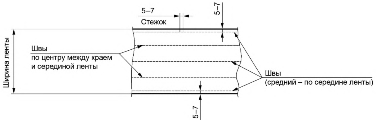
Рисунок 13 — Пятишовная сшивка
