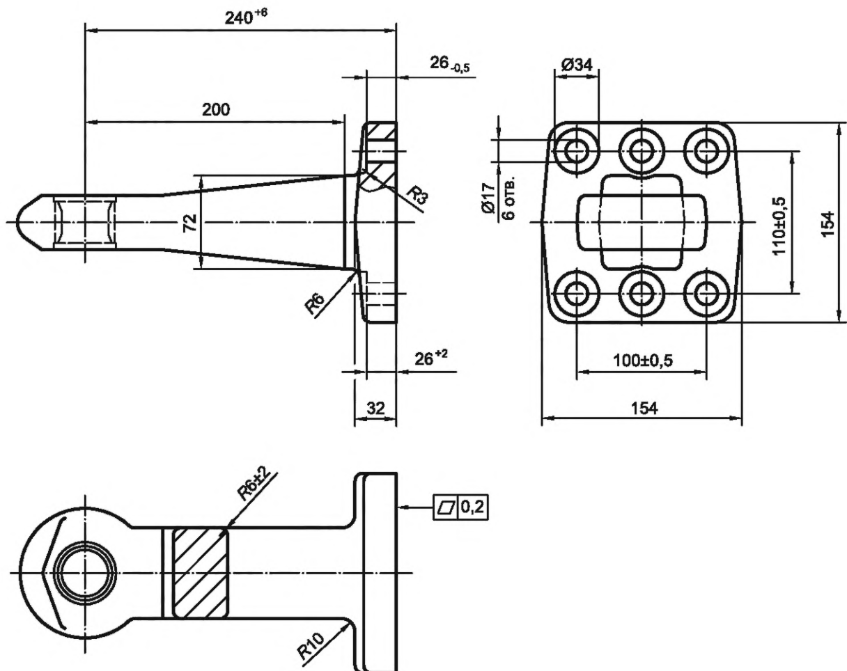
Рисунок А.12 — Конструкция и размеры сцепной петли неврещающейся с рельефной втулкой диаметром 40 мм, варианта В для элемента ТСУ «вилка вращающаяся»
