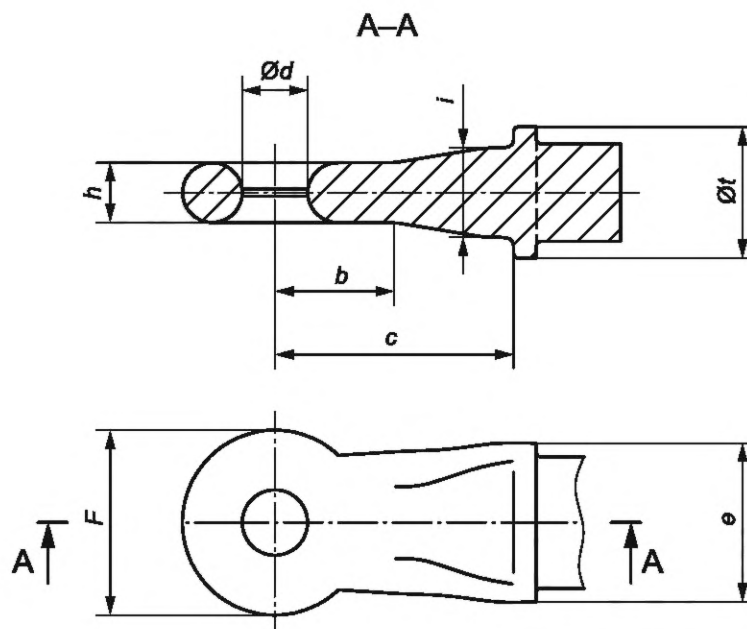
Рисунок А.14 — Конструкция и размеры сцепных петель вращающихся варианта W, X, Y или Z с круглым сечением тела проушины для элемента ТСУ «вилка неврещающаяся»
