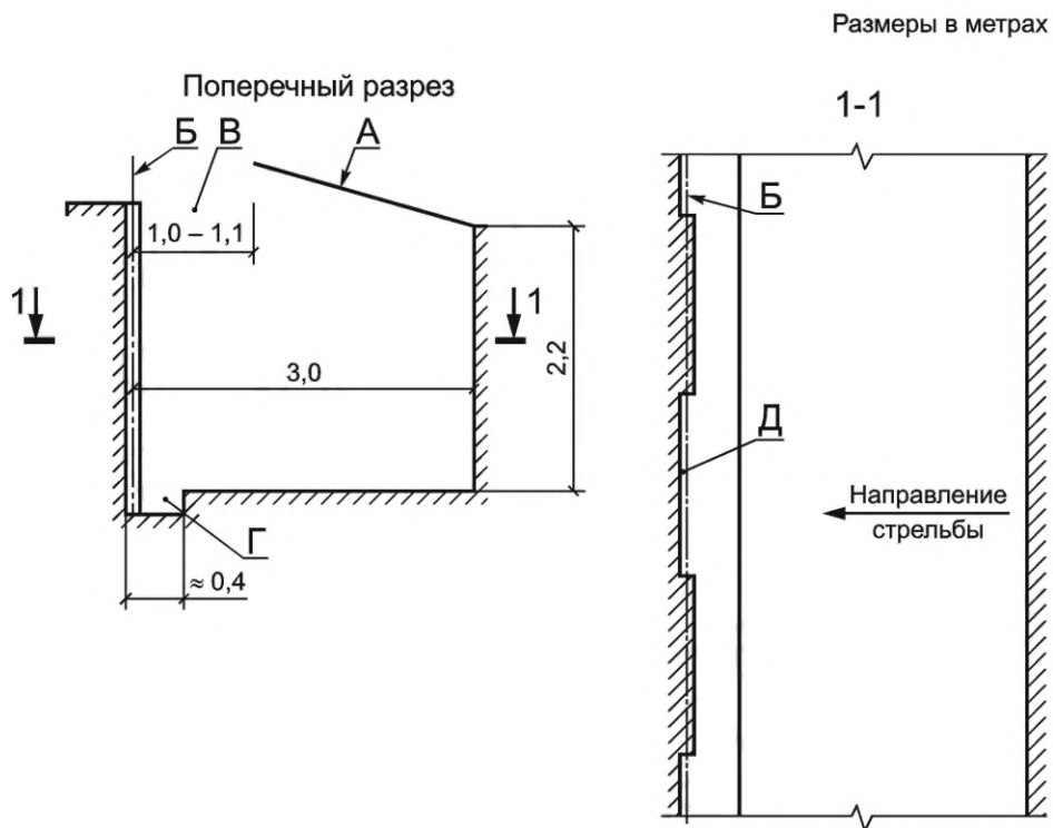
Рисунок Б.1 — Блиндаж огневой зоны крытого тира (вариант решения)
