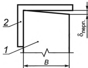
1 — панель; 2 — поверочный угольник 90^\circ ; B — ширина панели
