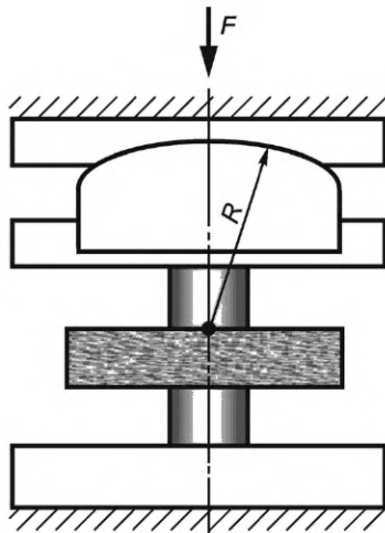
Рисунок А.2 — Схема испытаний с двухсторонним приложением нагрузки на образец через штампы
