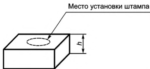
Рисунок 1 — Образец-пластина высотой h
