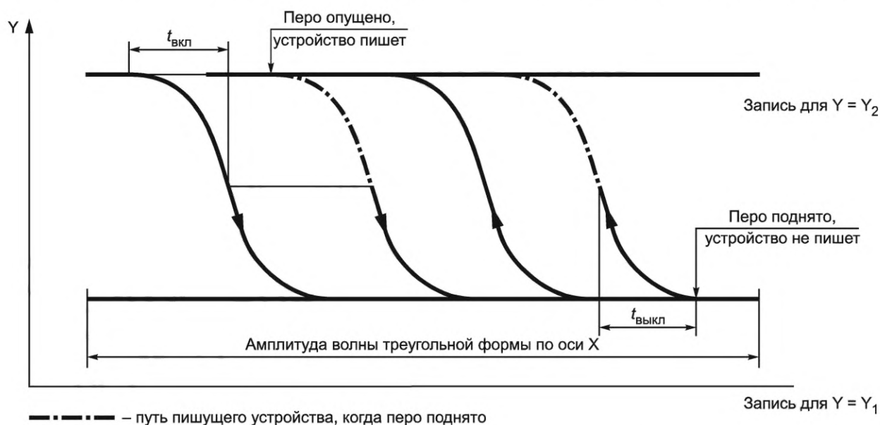
Рисунок 1 — Определение времени задержки для включения и выключения записи
