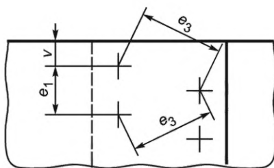
Рисунок 18 — Контактная точечная сварка листового металла, однорядная
