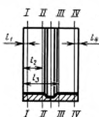
Вкладыш с кольцевой масляной канавкой
