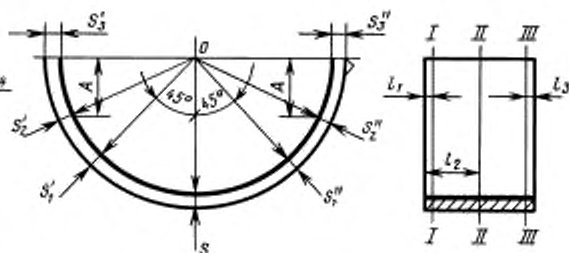
Вкладыш без масляной канавки
