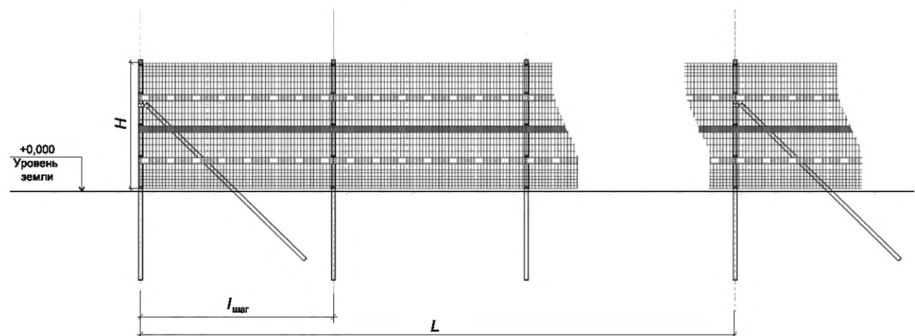
Рисунок 10 — Рулонно-секционное ограждение с типом полотна P2
