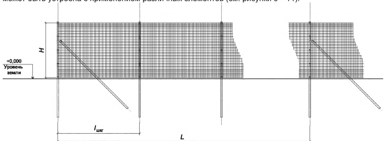
Рисунок 9 — Рулонно-секционное ограждение с типом полотна P1
