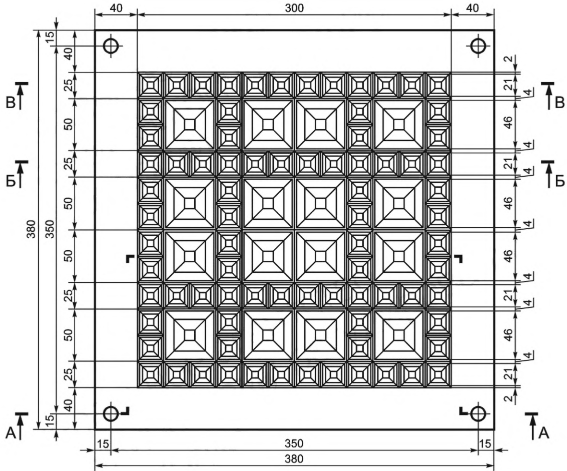
Рисунок А.1 — Щебеночная плита
