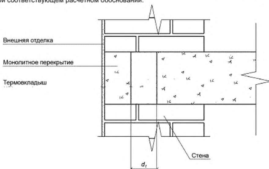
Рисунок 2 — Принципиальная схема устройства термовкладышей в монолитном диске перекрытия (разрез)
