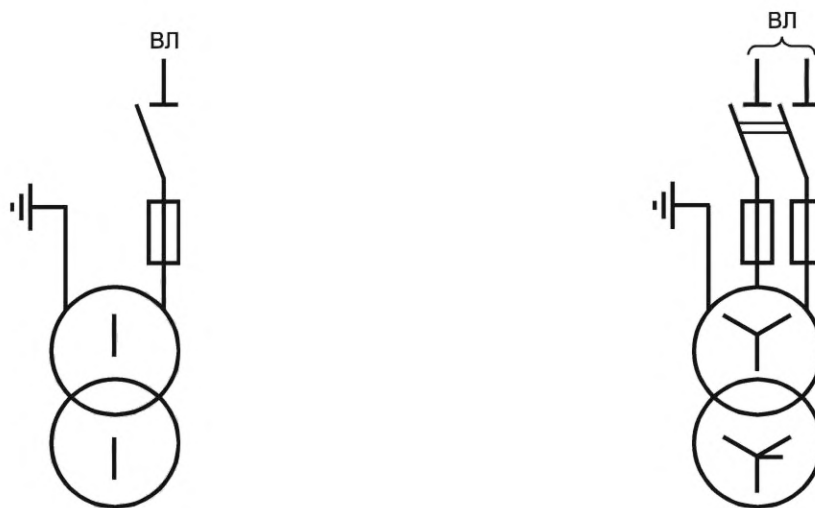
в) Схема для подстанций с высшим напряжением 27,5 кВ, воздушным вводом и однофазным трансформатором
