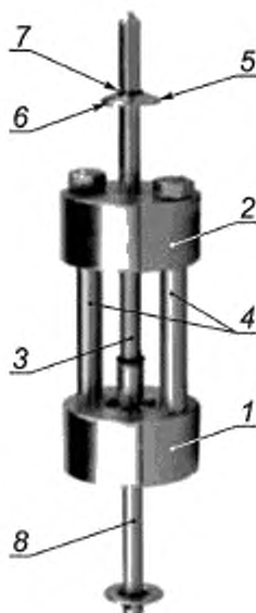
1 — основание, 2 — верхняя платформа; 3 — подвижной стержень, 4 — стойки-колонки; 5 — универсальная опора; 6 — кольцо; 7 — С-зажим; 8 — стержень-подвеска
