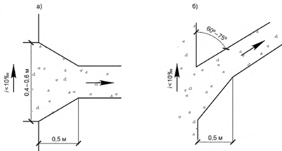
а) — примыкание воронки к песчаному слою при малых уклонах; б) — то же при уклоне более 10 ‰
