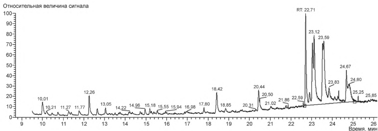
Рисунок А.2 — Типовая хроматограмма градуировочного раствора СуcDs с массовой концентрацией 25 мг/дм 3
