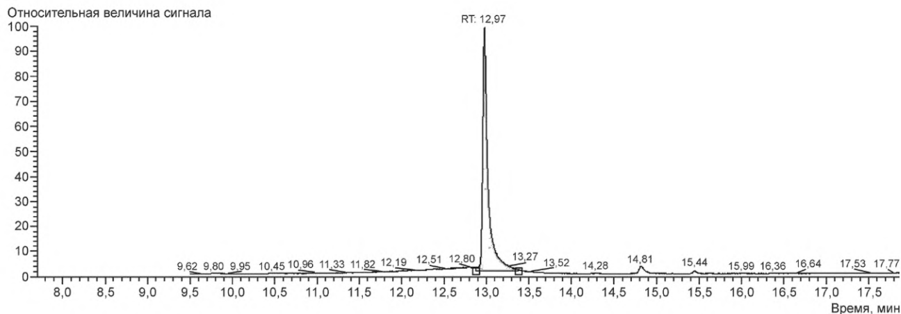
Рисунок А.1 — Типовая хроматограмма градуировочного раствора 3-MPD с массовой концентрацией 25 мг/дм 3
