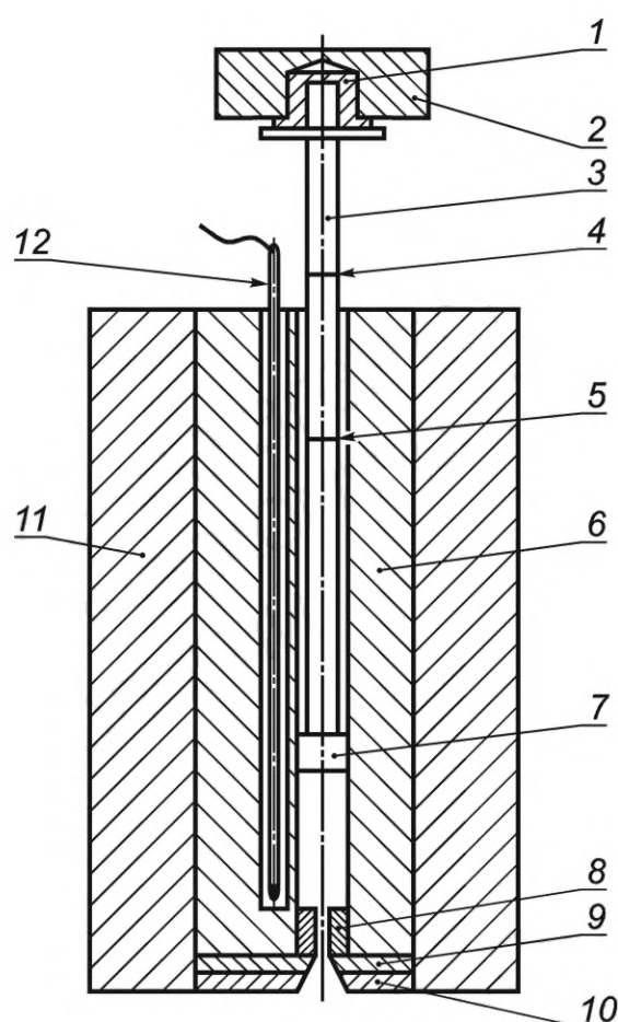
1 — теплоизоляция; 2 — съемный груз; 3 — поршень; 4 — верхняя контрольная метка; 5 — нижняя контрольная метка; 6 — эструзионная камера; 7 — направляющая головка поршня; 8 — капилляр; 9 — пластина, удерживающая капилляр; 10 — изолирующая пластина; 11 — теплоизоляция; 12 — датчик температуры
