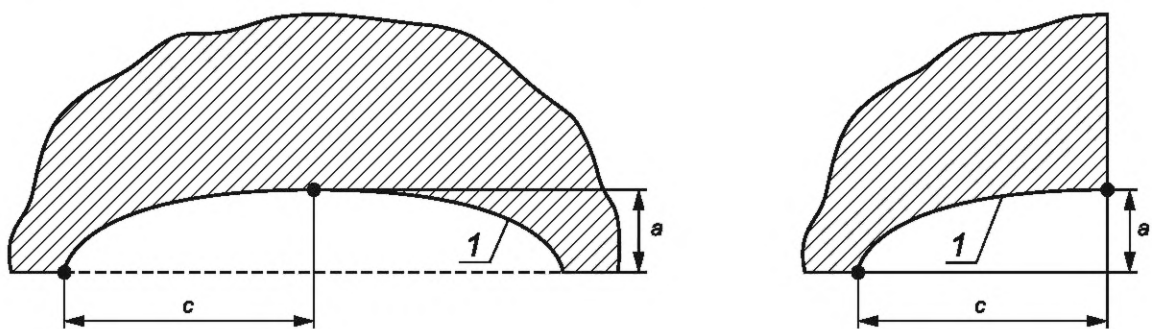
а) Поверхностная полуэллиптическая трещина
