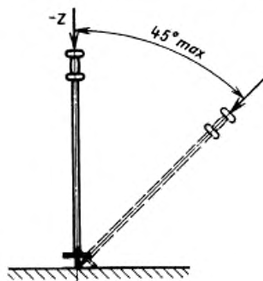
Схема испытания на сцепление наконечника со льдом
