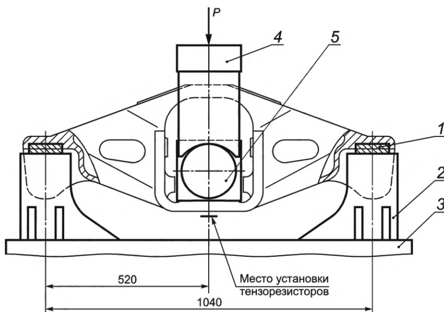
1 — вкладыш; 2 — опора; 3 — стол испытательного стенда; 4 — П-образное приспособление; 5 — брус с цилиндрическими концевыми частями
